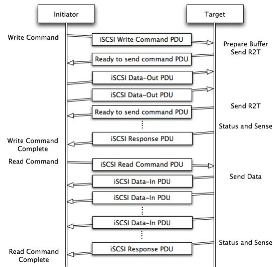
圖 1. iSCSI 之讀寫操作
