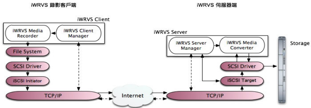
圖 3. 影像寫入之架構圖
