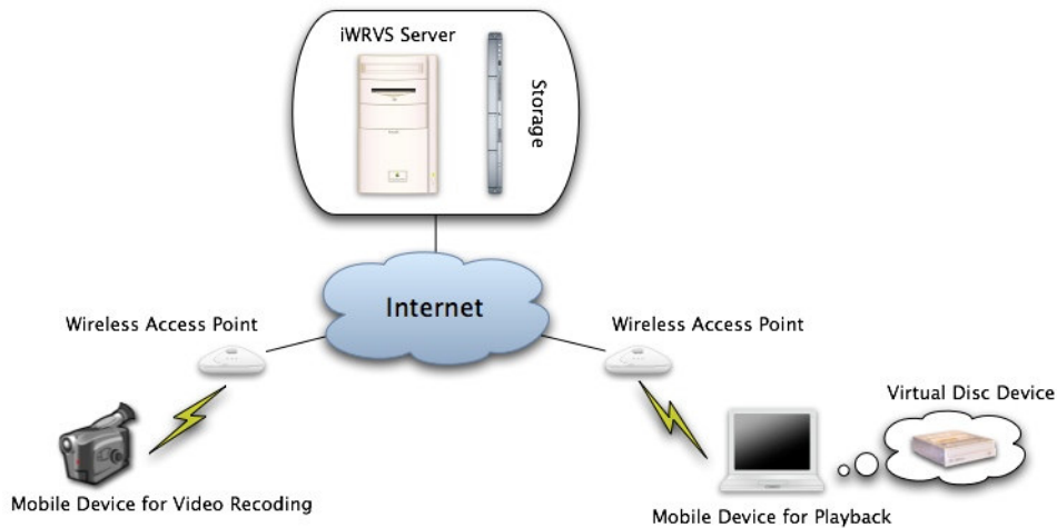
圖 2. iWRVS 系統示意圖
