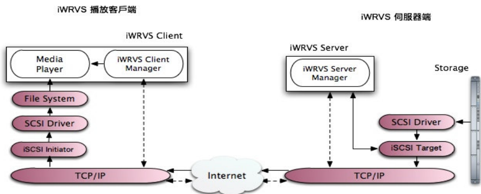
圖 5. 影像播放之架構圖
